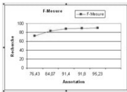
Figure 5 : Evolution des résultats de la recherche par rapport à celles de l'annotation
