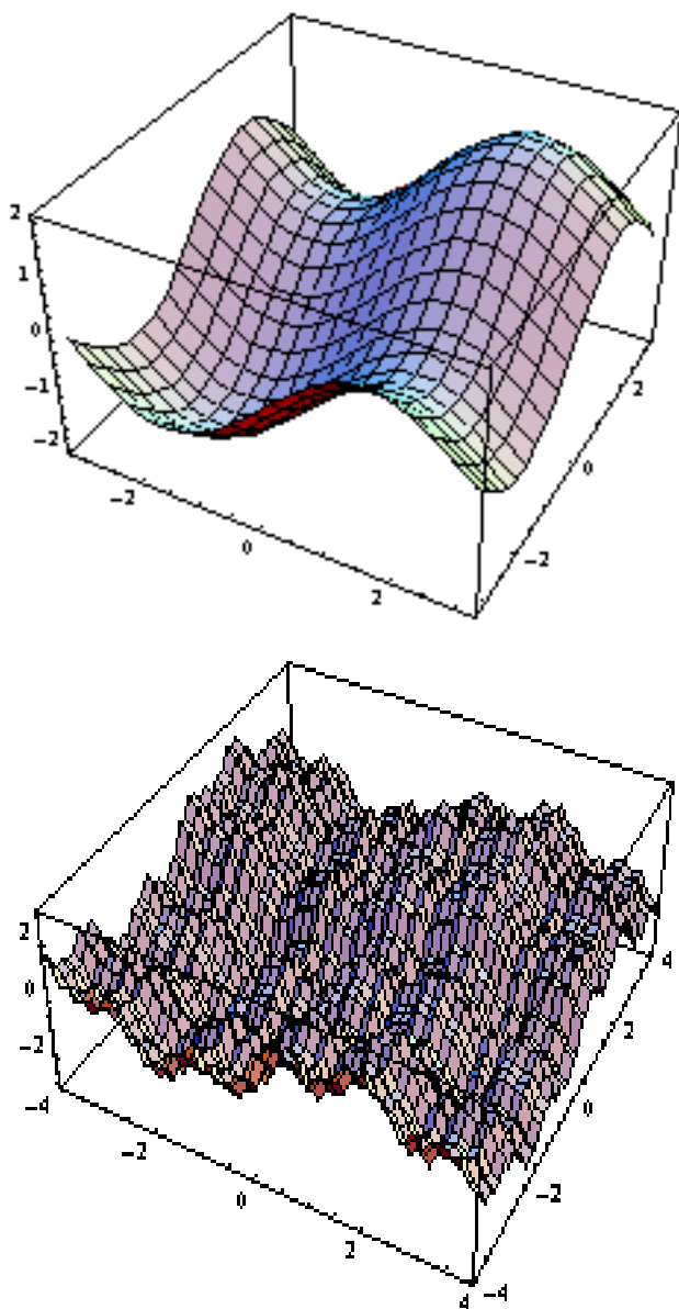
Fig 2: Espace courbe (en haut) et espace fractal (en bas) (d'après Nottale, 2002).
