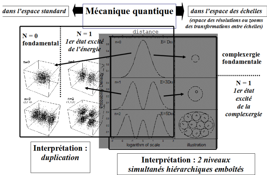
Fig 4: Les effets de la relativité d'échelle en mécanique quantique dans l'espace standard et l'espace des échelles.
